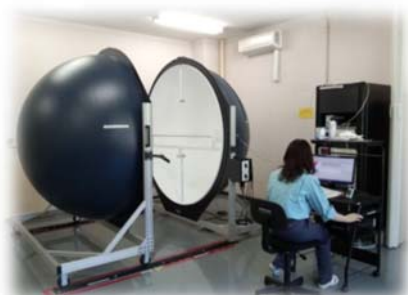
全光束試験
